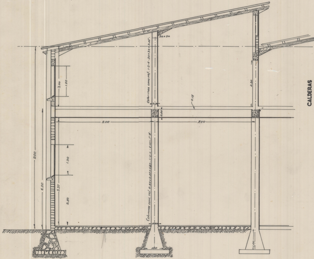
SECCION SEGUN LA LINEA "A-A" DE LA PLANTA ANEXA (Secc. vert. Long). ESCALA, 1:50.
