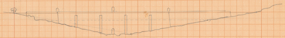
SECCION LONGITUDINAL DE LA CORTINA E/SCALA 1:1000
