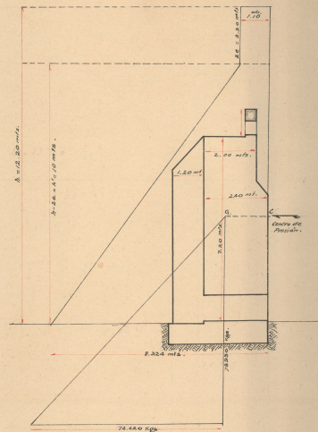
CORTE DE LA CORTINA, ESC 1:100
