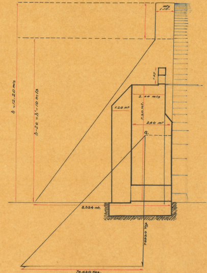
CORTE DE LA CORTINA. ESC. 1:100
