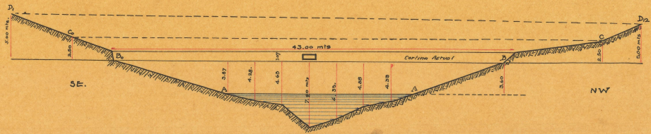
PERFIL DE LA CORTINA. ESCALA. 1:250 VERT. Y HOR.
