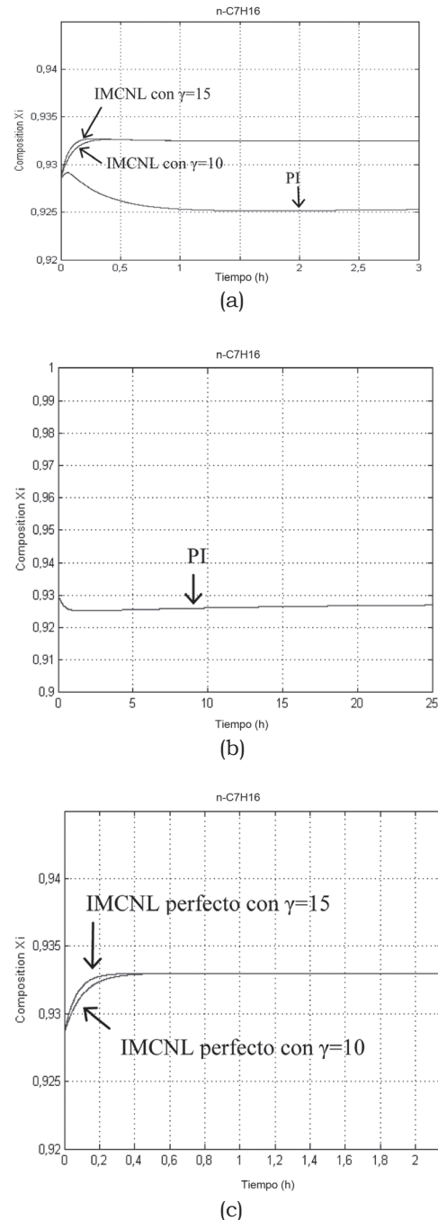
Figura 11. Cambio escalón en el set\text{-point} de la composición de B a x_{3B}=0,9330 (cambio +0,46 %). a) Comparación de los controladores IMCNL imperfectos y PI; b) respuesta dinámica del controlador PI; c) respuesta dinámica del controlador IMCNL perfecto.
