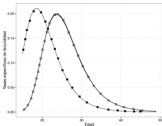
Figura 3. Comparativo entre tasas específicas de fecundidad pronosticadas al año 2014 (-) con intervalos de predicción del 95% (+), respecto a las obtenidas en la Encuesta Nacional de la Dinámica Demográfica 2014. Fuente: Cálculos propios con base en Somede (2011) y INEGI (2015).
