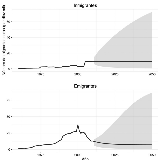
Figura 5. Migración internacional femenina estimada 1950-2010 y pronosticada 2011-2050 (línea negra) con intervalos de predicción del 95% (franja gris). Fuente: Cálculos propios con base en Somedé (2011).
