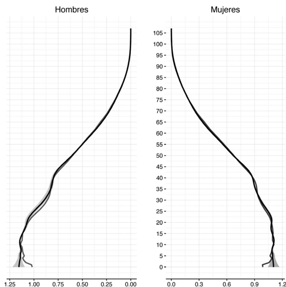
Figura 7. Distribución por edad y sexo para la población estimada 1950-2010, pronosticada 2011-2050 (curvas negras) con intervalos de predicción del 95% (franja gris claro) y estimada al 2015 de acuerdo a la Encuesta Intercensal 2015 (curva gris). En millones. Fuente: Cálculos propios con base en Somede (2011) y INEGI (2016).
