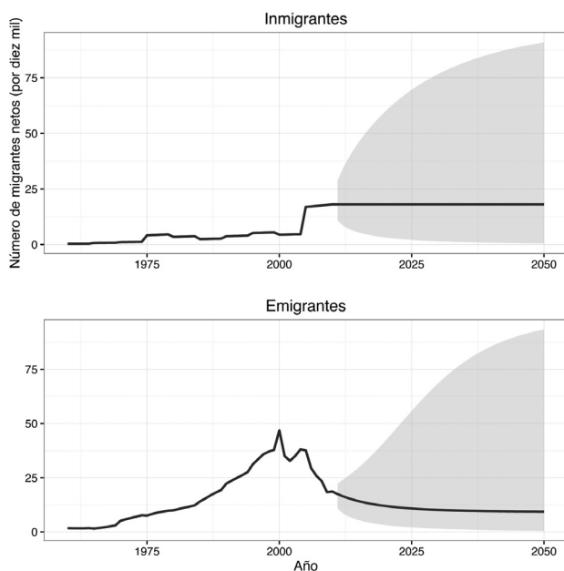
Figura 4. Migración internacional masculina estimada 1950-2010 y pronosticada 2011-2050 (línea negra) con intervalos de predicción del 95% (franja gris). Fuente: Cálculos propios con base en Somedé (2011).
